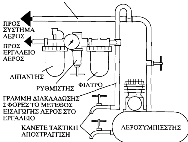
ΚΥΡΙΕΣ ΓΡΑΜΜΕΣ 3 ΦΟΡΕΣ ΤΟ ΜΕΓΕΘΟΣ ΤΗΣ ΕΙΣΑΓΩΓΗΣ ΑΕΡΟΣ ΣΤΟ ΕΡΓΑΛΕΙΟ
